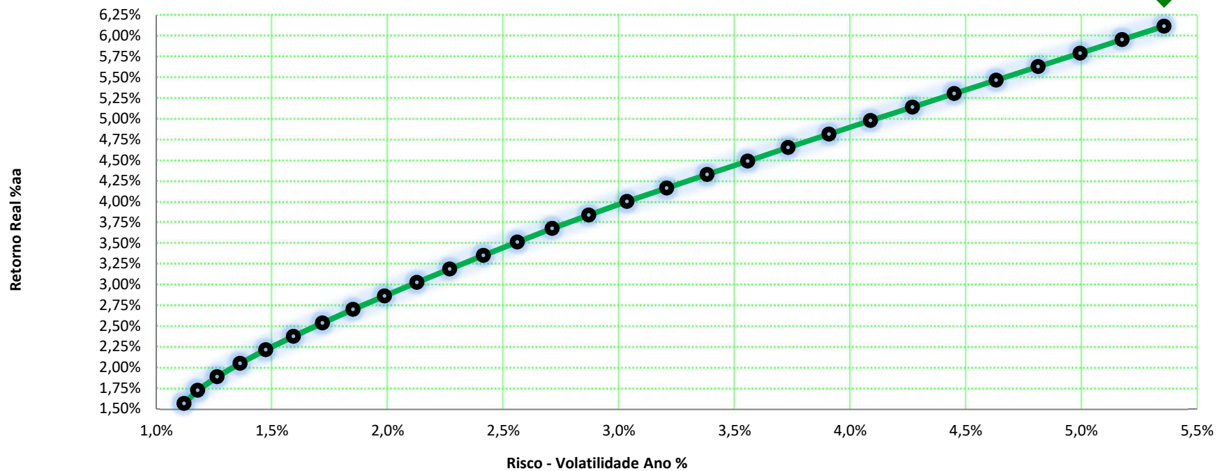
Fronteira Eficiente de Markowitz
